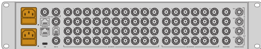
Микшер ATEM 4 M/E Constellation HD оснащен дополнительным силовым входом по стандарту IEC
