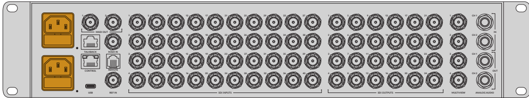
ATEM 4 M/E Constellation HD, yedeklik için ikinci bir IEC güç girişine sahiptir
