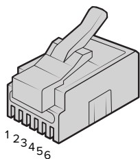
ATEM 4 M/E Constellation HD上PTZ遥控的RJ12引脚示意图
