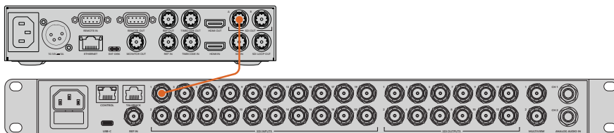
将HyperDeck Studio HD Plus的SDI输出连接到ATEM 2 M/E Constellation HD的SDI输入。
