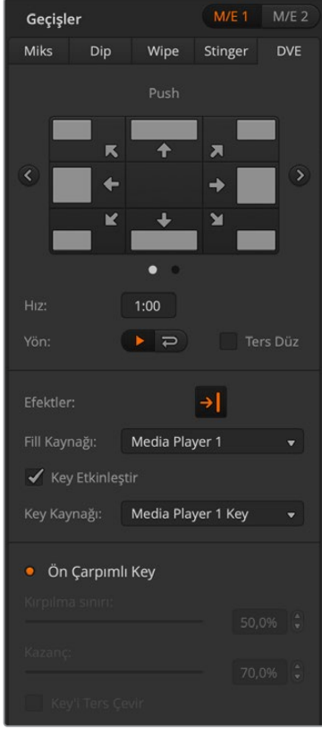
DVE Geçiř Ayarları
