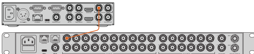
Collega l'uscita SDI di Hyperdeck Studio HD Plus a un ingresso SDI di ATEM 2 M/E Constellation HD
